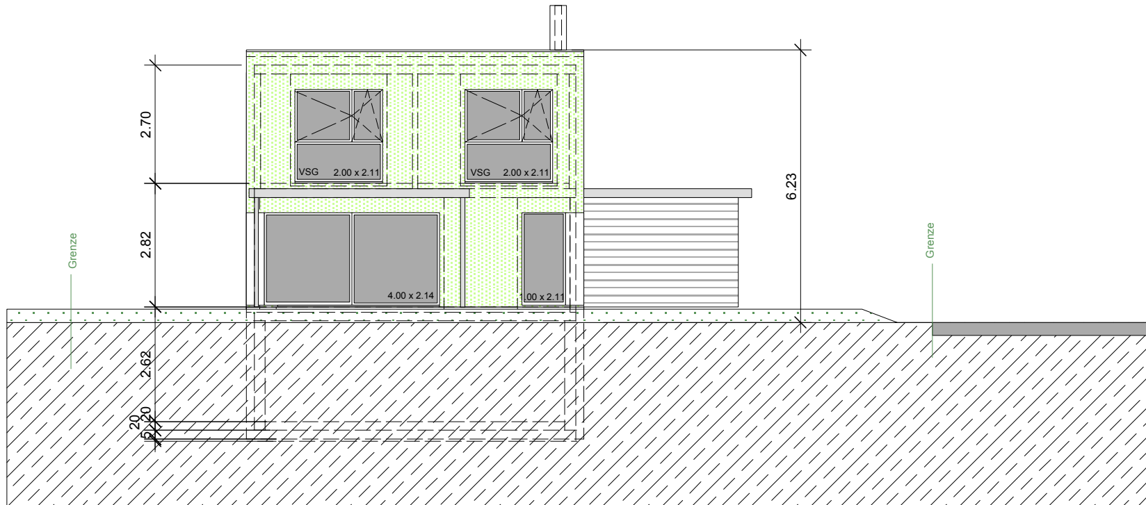
Süd - Westansicht
