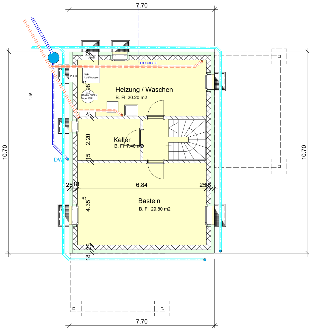
Grundriss Untergeschoss
