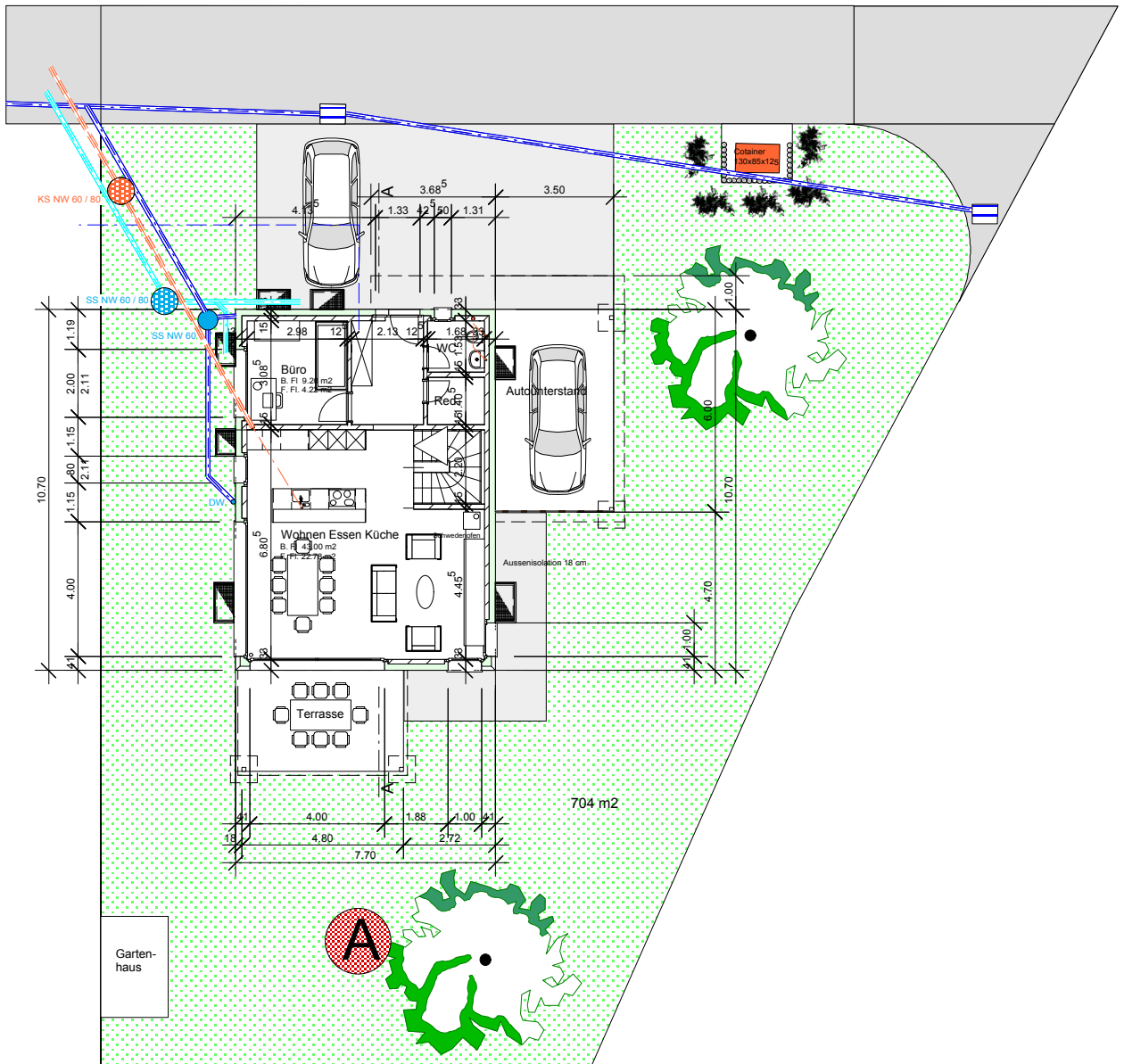
Grundriss Erdgeschoss
