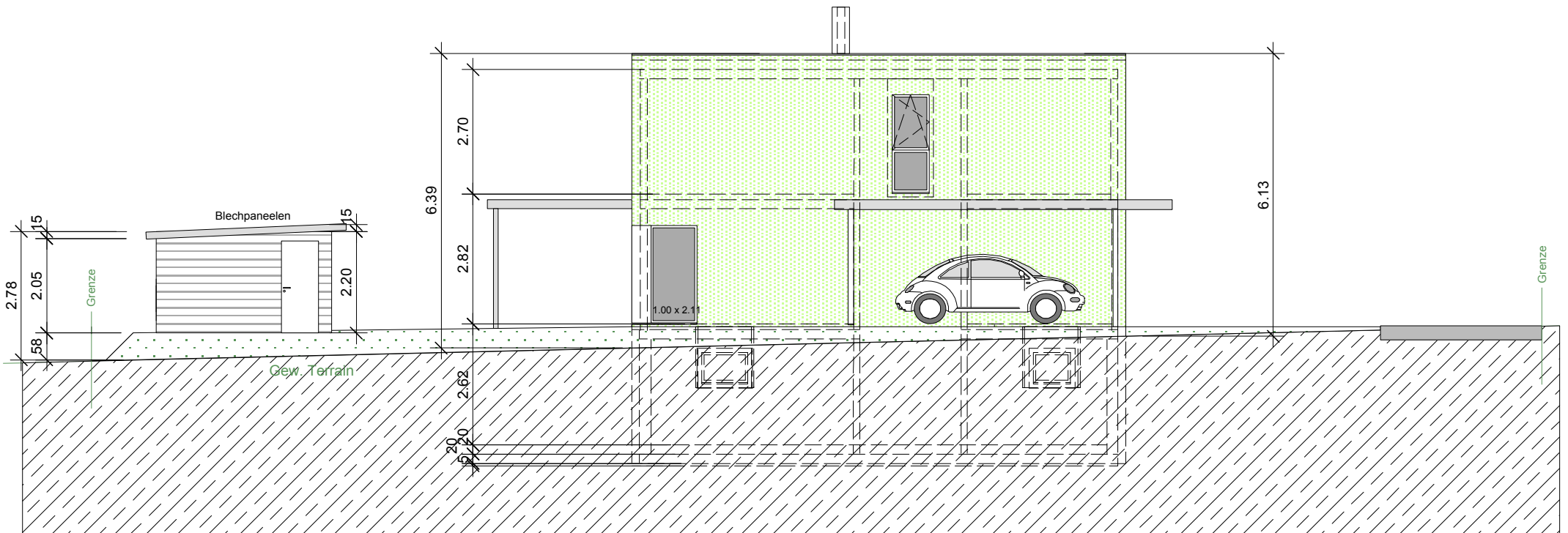
Süd - Ostansicht
