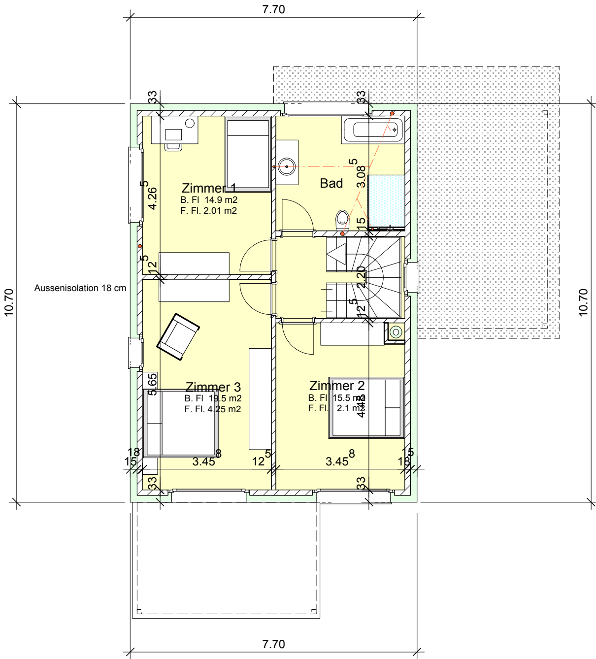
Grundriss Obergeschoss
