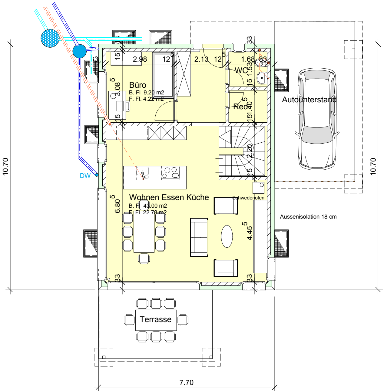
Grundriss Erdgeschoss
